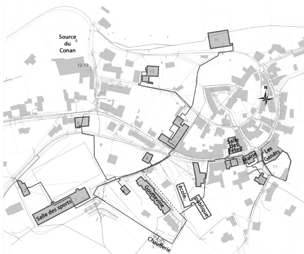
Tracé du réseau de chaleur de Montrottier
